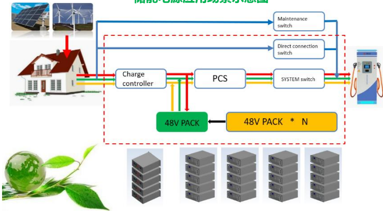
储能电源应用场景示意图
